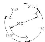
Bohrbild Deckel
